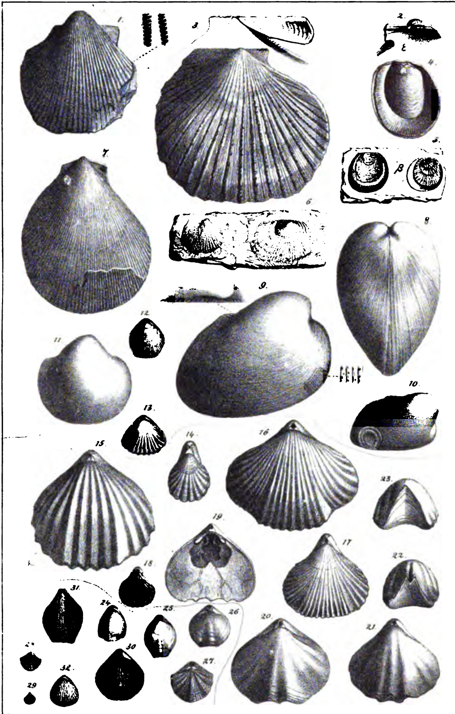
Lucasella Lucasella
